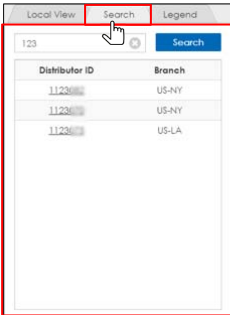
Search Module
