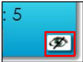
Hide Icon
