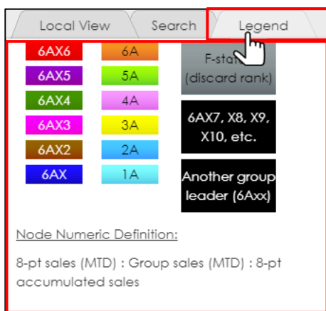
Legend Module
