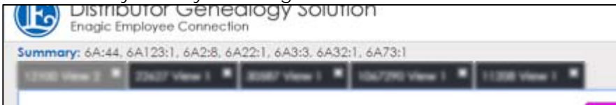
Tabs
